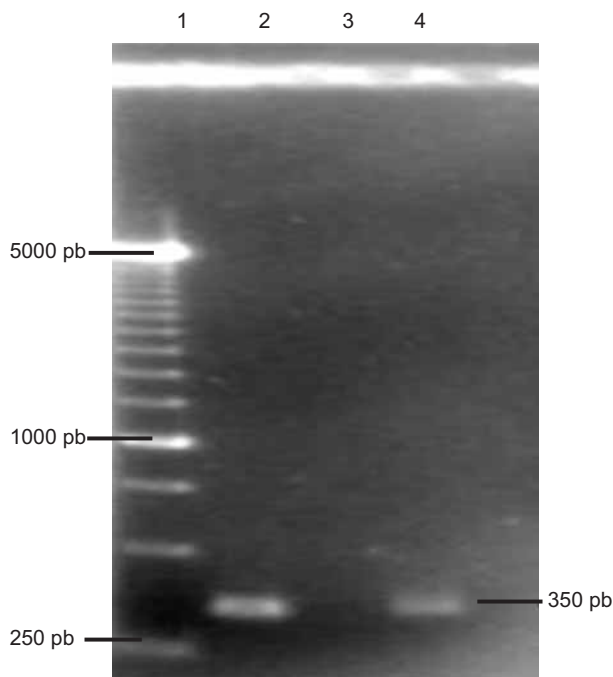
Figura 1 | Productos de la PCR de Trypanosoma cruzi . Carril 1, marcador de peso molecular de 250 pb; carril 2, muestra; carril 3, control negativo (agua); carril 4, control positivo (cepa Ninao)
